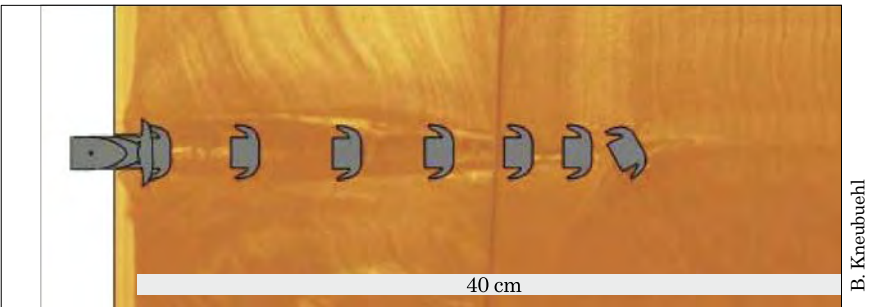
図 3.23 石鹼塊の中で変形する拳銃用弾丸。マッシュルーム化が見られる (弾丸の動きを石鹼塊に重ねた図)。
