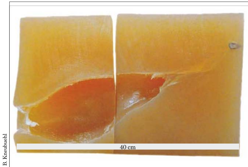
写真 3.21 石鹼塊を用いて、跳弾効果を伴うライフル用 FMJ 弾が与える影響を示す。安定性を失った跳弾は、早期から容易に回転運動を始め、大きな接触面をもって着弾する。SJ 弾と同様に、ほぼ着弾直後から空洞を形成する。
