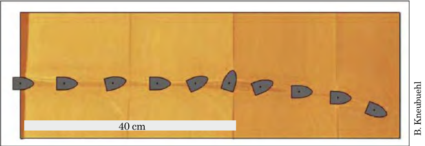
図 3.22 石鹼塊を用いて、標準的な軍用ピストル弾 (FMJ) の動きを示す。回転は伴わないことがわかる (弾丸の動きを石鹼塊に重ねて図式説明する)。
